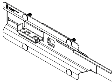
Combo Latch No Bezel
