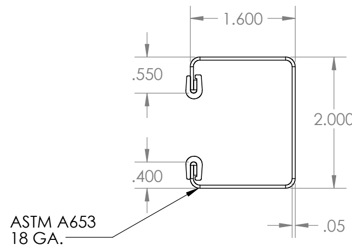
DOOR GUIDE DETAIL
