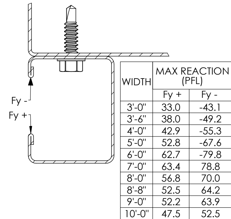
DOOR GUIDE FORCE
