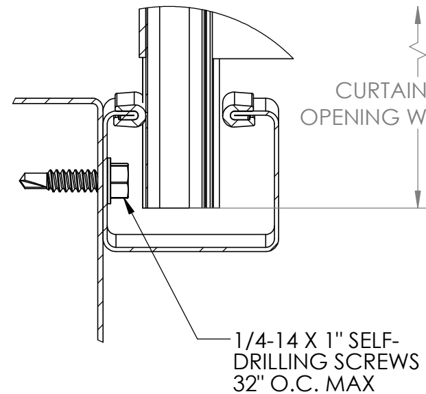
DOOR GUIDE TO STEEL JAMB
